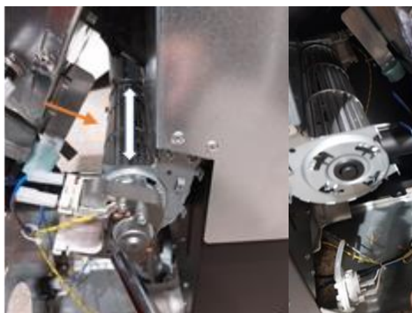
Rys. 45 - Czyszczenie wentylatora otoczenia
